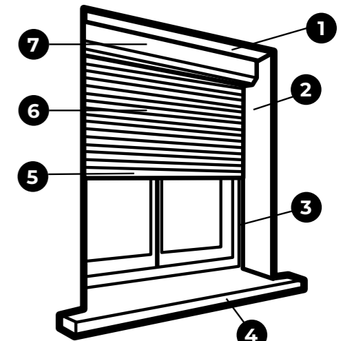
1 Linteau 2 Tableau 3 Coulisserie 4 Appui 5 Lame finale 6 Tablier 7 Coffre
